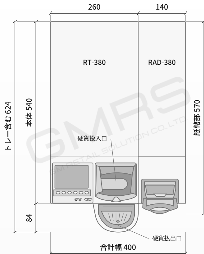
上面図
