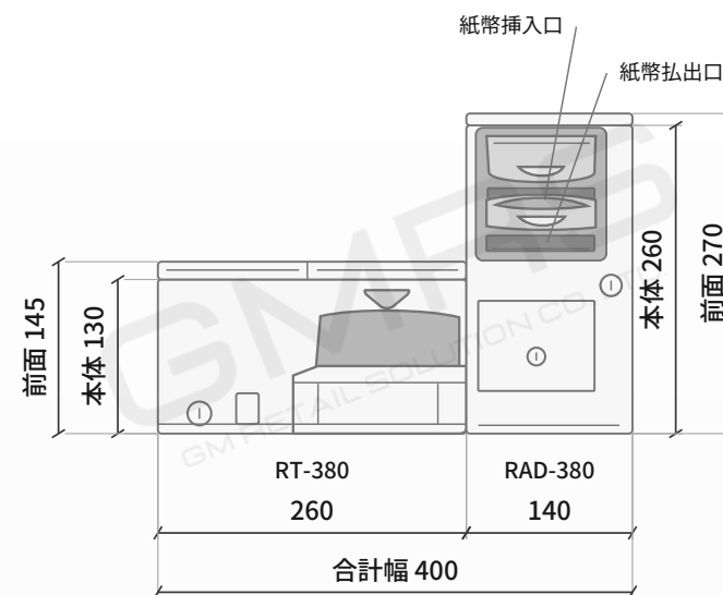
正面図
